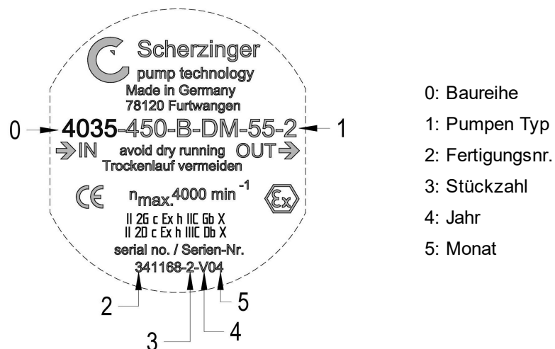
Abb. 1: Typenschild zu Pumpe mit Motor
