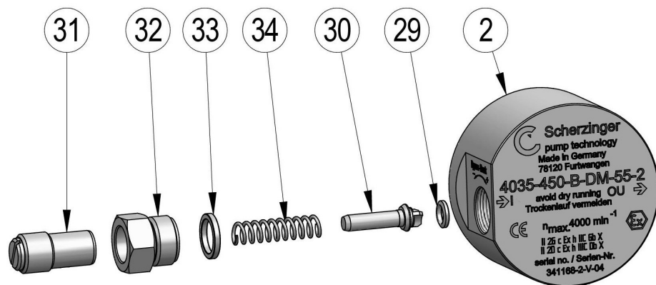
Abb. 6: Druckbegrenzungsventil
