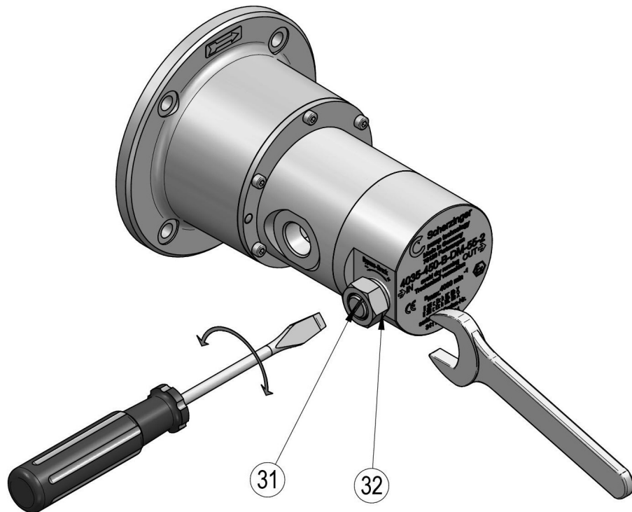
Abb. 7: Einstellung des Druckbegrenzungsventils
