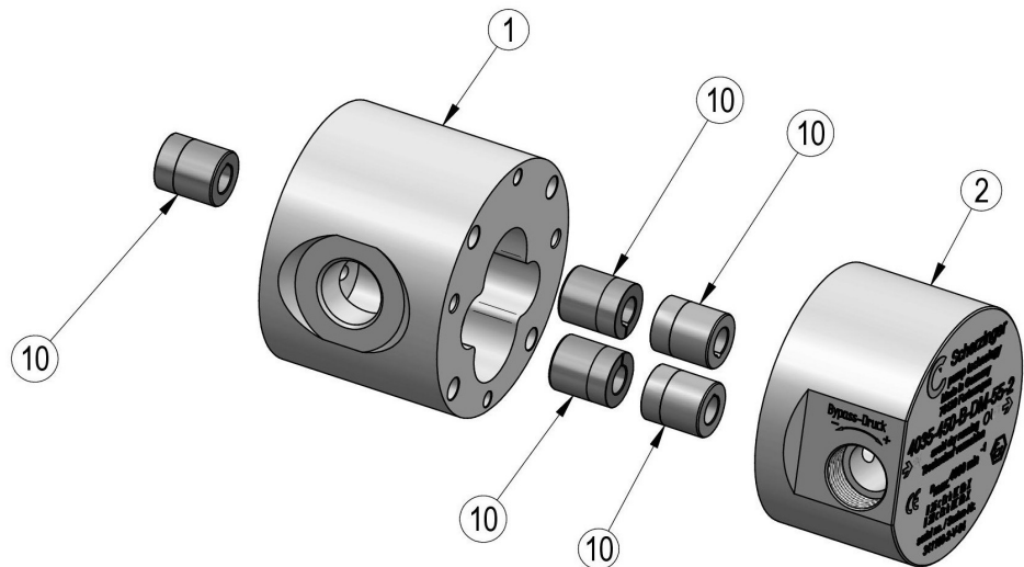
Abb. 9: Wellenlager
