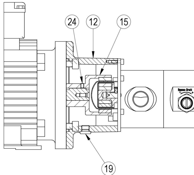
Abb. 10: Montage der Magnetkupplung
